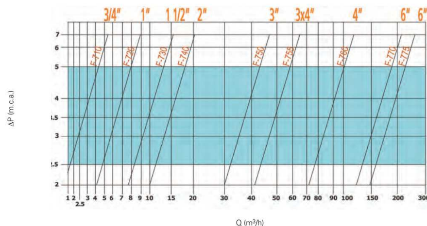
PORTATE E PRESSIONI MASSIME
