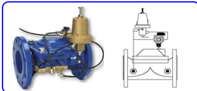
VALVOLA DI SOSTEGNO PRESSIONE DI MONTE CON PILOTA A 3 VIE
