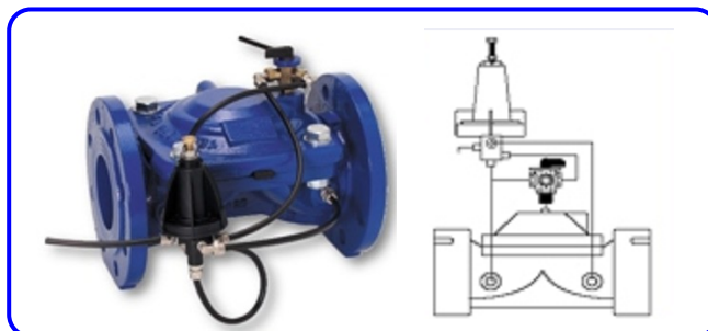
VALVOLA RIDUTTRICE DI PRESSIONE CON PILOTA A 3 VIE.
