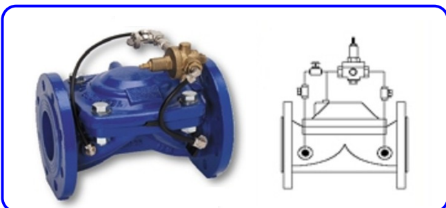
VALVOLA RIDUTTRICE DI PRESSIONE CON PILOTA A 2 VIE.
