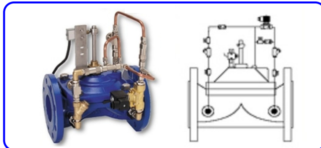
VALVOLA DI CONTROLLO POMPA.
