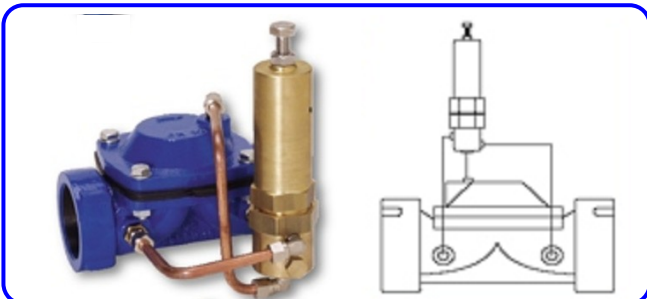
VALVOLA DI SCARICO RAPIDO CONTRO IL COLPO DI ARIETE.
