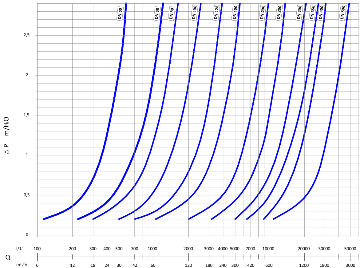
DIAGRAMMA PERDITE DI CARICO - HEAD LOSS DIAGRAM
